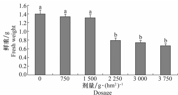
图2 50%异丙隆 WP 对小麦地上部鲜重的影响
