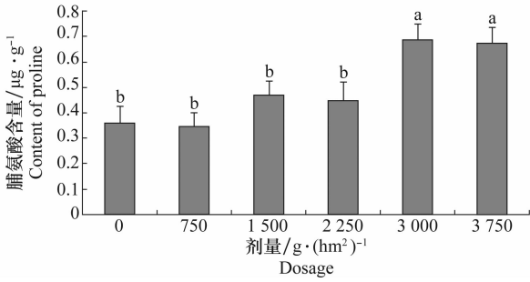
图 7 50%异丙隆 WP 对小麦 Pro 含量的影响
