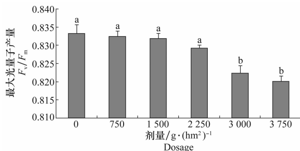
图4 50%异丙隆 WP 对小麦 F_v/F_m 的影响
