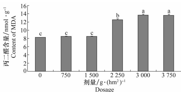
图5 50%异丙隆 WP 对小麦 MDA 含量的影响
