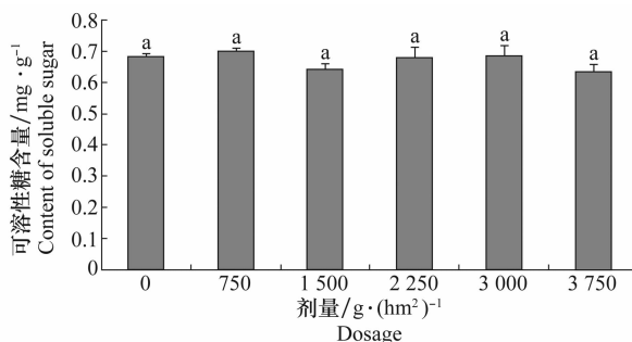
图6 50%异丙隆 WP 对小麦可溶性糖含量的影响
