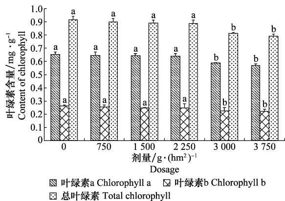
图3 50%异丙隆 WP 对小麦叶绿素含量的影响
